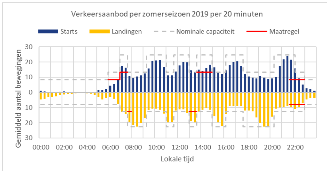
Figuur 4: Gecombineerd effect van het verlengen van het nachtrechtime en het verminderen van het gebruik van secundaire banen op de beschikbare afhandelingscapaciteit, ten opzichte van het verkeersbeeld van het zomerseizoen in 2019.
